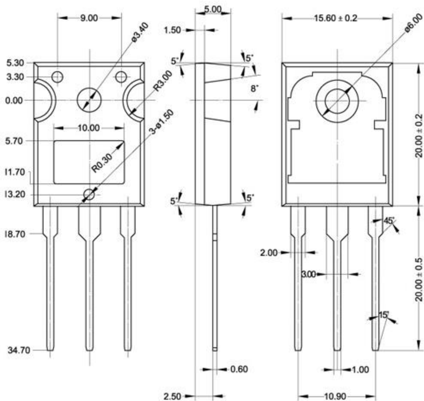
Габаритный чертёж корпуса КТ-43В
